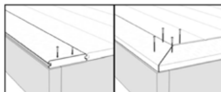
Instalación estándar Instalación en disposición de marco
